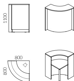
Lada narożna wysoka, łukowa H:1100 mm
