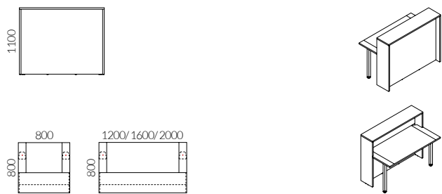
Lada prosta wysoka H:1100 mm
