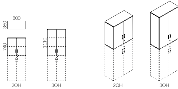
Nadstawka szafka z drzwiami skrzydłowymi Op-Lite
