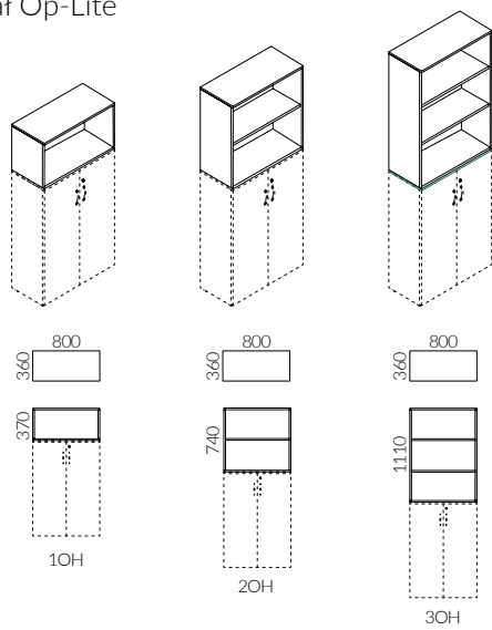
Nadstawka regał Op-Lite
