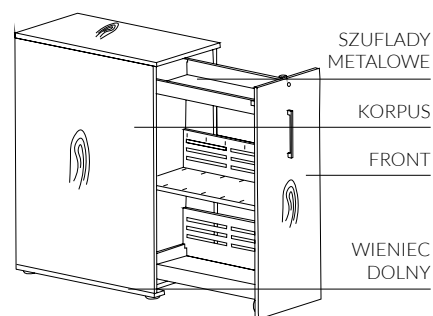
Kontener Cargo
