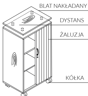
Kontener żaluzjowy
