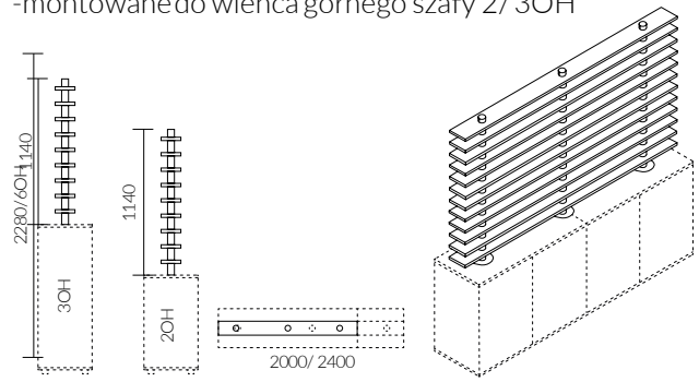
Diviso 3OH z trzema słupkami -montowane do wieńca górnego szafy 2/3OH
