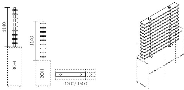
Diviso 3OH z dwoma słupkami -montowane do wieńca górnego szafy 2/3OH
