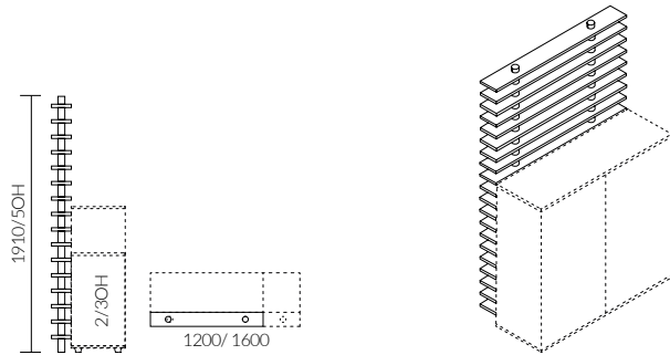
Diviso 5OH z dwoma słupkami -montowane do ściany tylnej szafy
