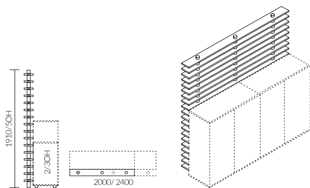
Diviso 5OH z trzema słupkami -montowane do ściany tylnej szafy
