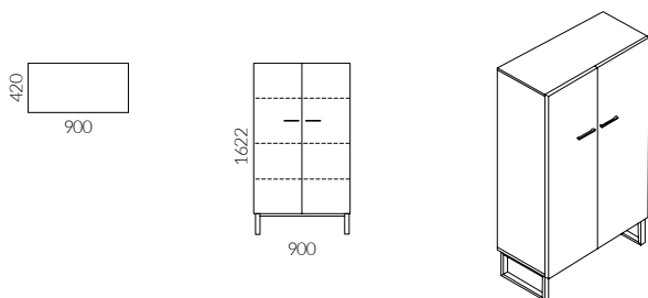
Szafa wysoka AXY-Line
