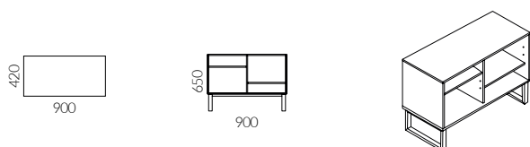
Szafa niska AXY-Line, otwarta
