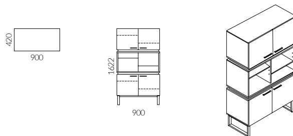
Szafa wysoka AXY-Line z otwartą częścią środkową
