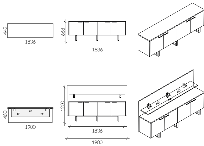
Witryna gabinetowa wąska AXY-Line
