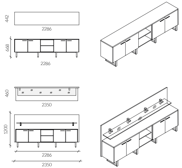
Witryna gabinetowa szeroka AXY-Line z częścią otwartą
